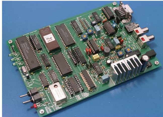
MuP-FAX CUBE51に組み込まれている切り替え回路の基板、リレー5個が使用されている。
